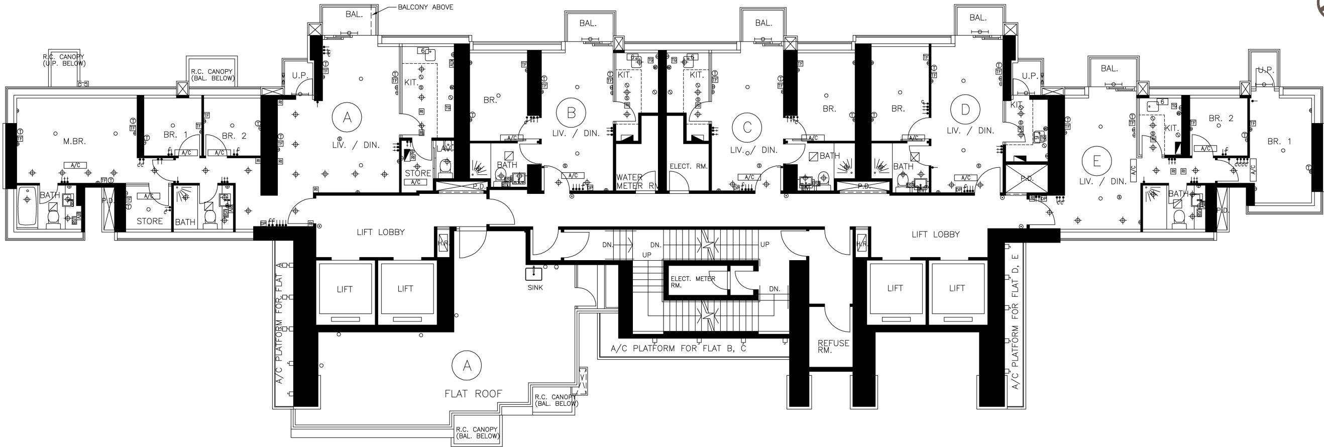
16/F Floor Plan 16樓平面圖
